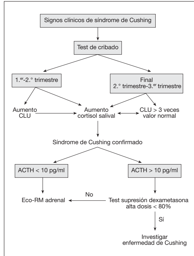
Fig. 1. Algoritmo de sospecha de síndrome de Cushing en el embarazo. ACTH: corticotropina; CLU: cortisol libre urinario; RM: resonancia magnética.
